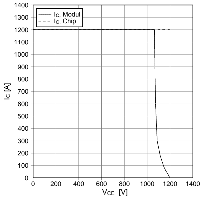
Sicherer Rückwärts-Arbeitsbereich IGBT-Wr. (RBSOA) reverse bias safe operating area IGBT-inv. (RBSOA) I_C = f(V_{CE}) V_{GE} = \pm 15\text{ V} , R_{Goff} = 1.2\ \Omega , T_{vj} = 125^\circ\text{C}
